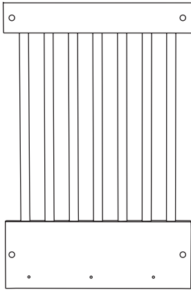
A-1. Left End Panel A-1 Panneau latéral gauche
